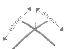
Base a croce grande UF-ZMLCB
